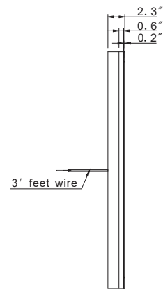
LEFT SIDE
